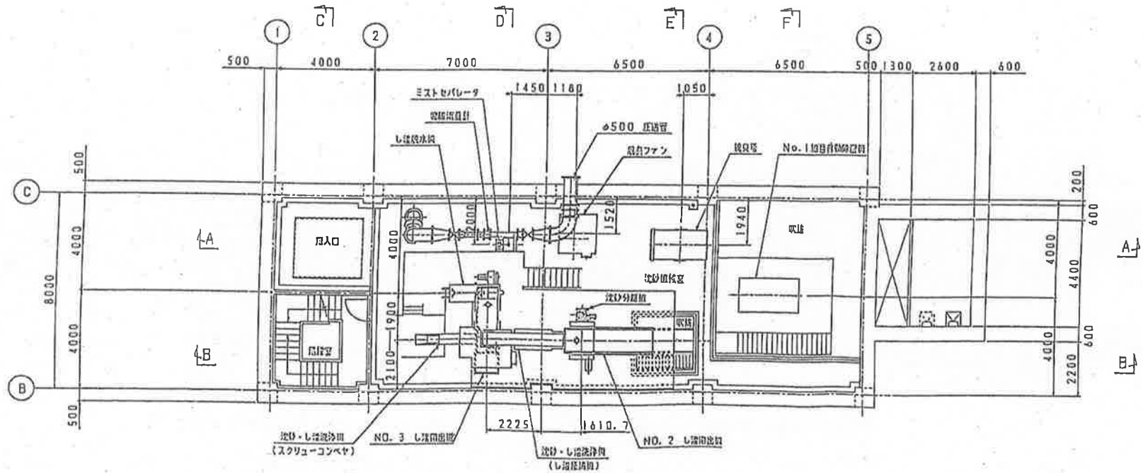
悪臭測定箇所(脱臭設備)
